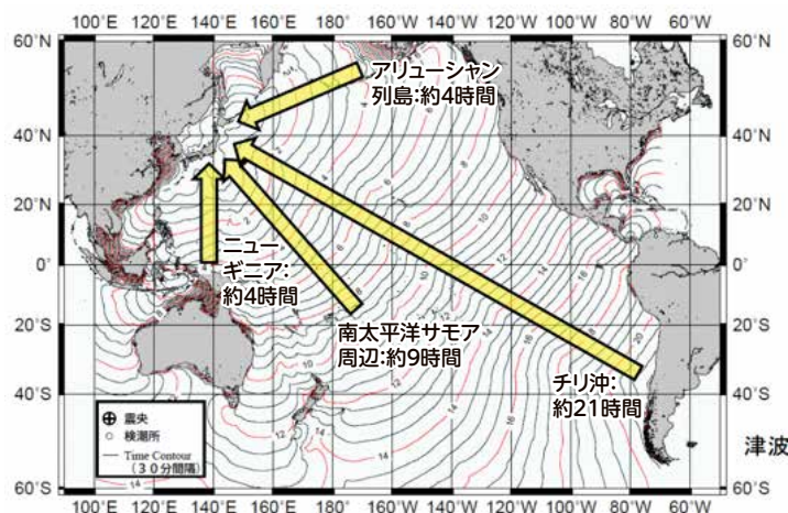
日本への遠地津波到達時間
