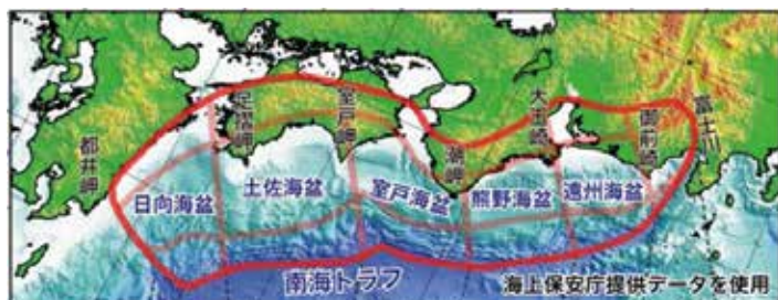
南海トラフ地震震源域
