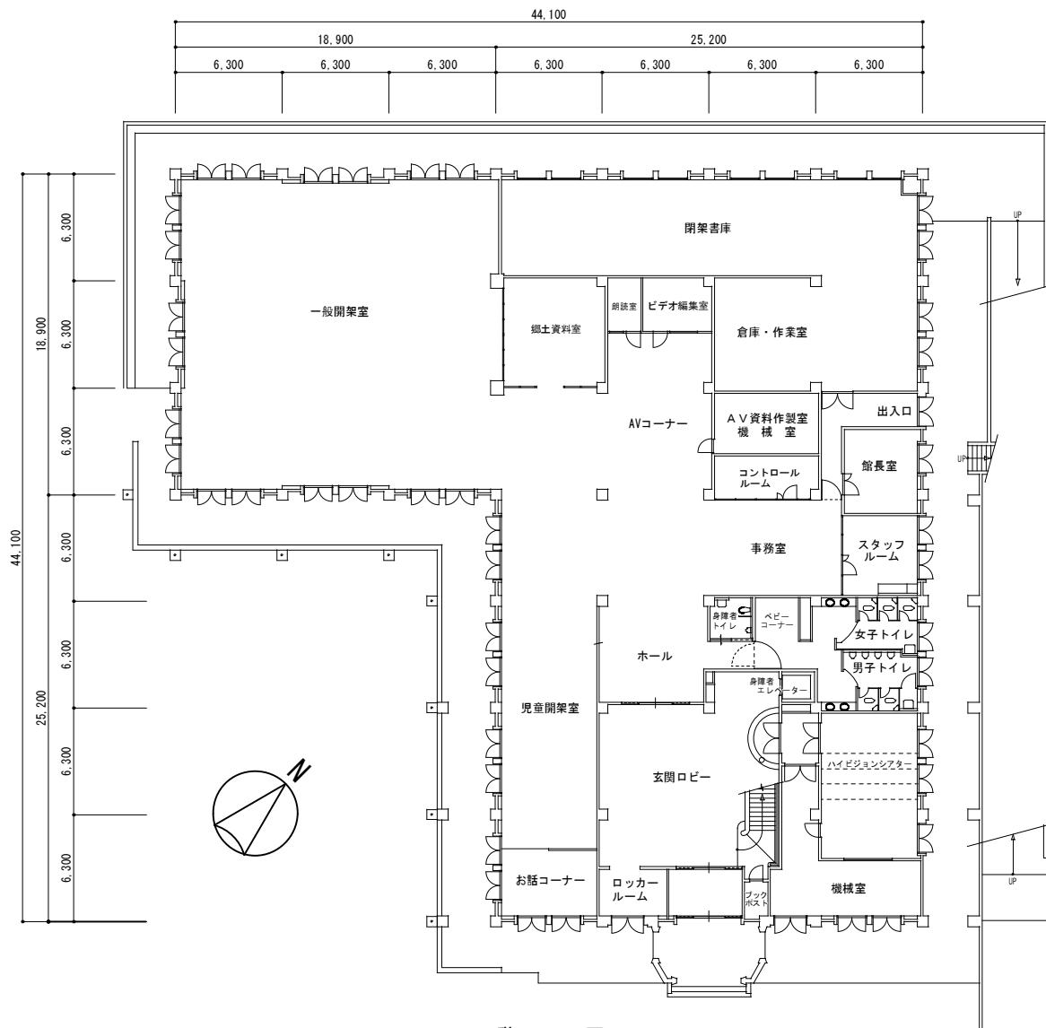
1階平面図
