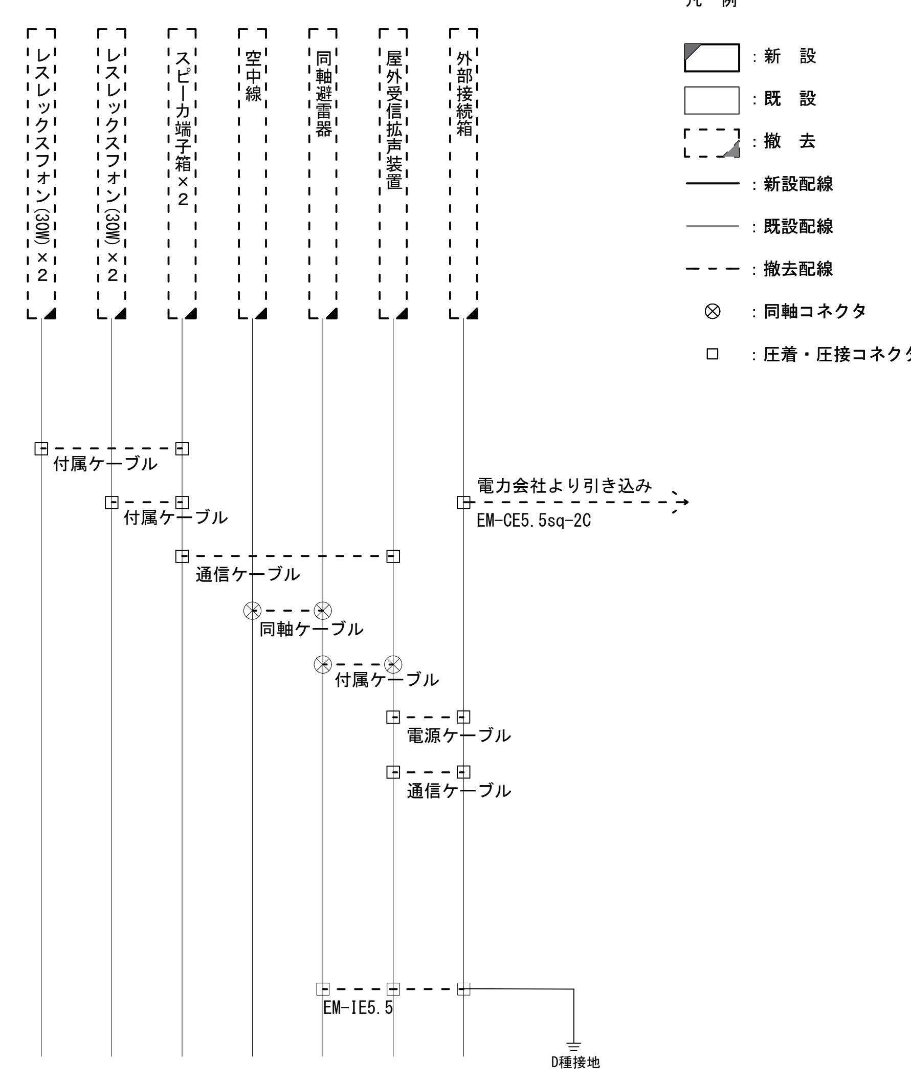
配線系統図
