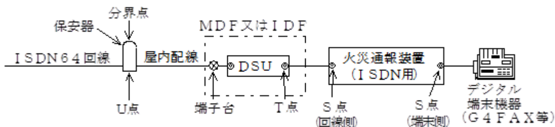
第14-4図（火災通報装置（ISDN用）とISDN64回線の接続例）
