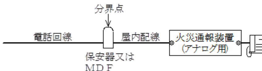
第14-2図（P B X等がない場合）
