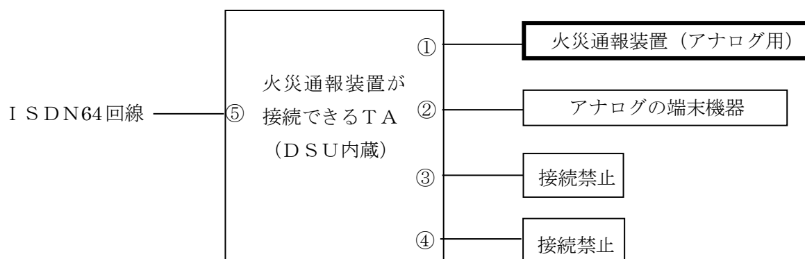
第14-5図 b（TAにDSUが内蔵されている場合の各接続端子の接続例）
