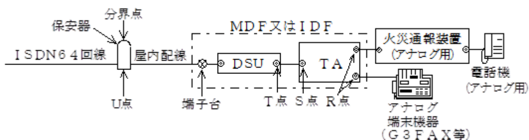
第14-5図 a（火災通報装置（アナログ用）をISDN64回線に接続する場合）
