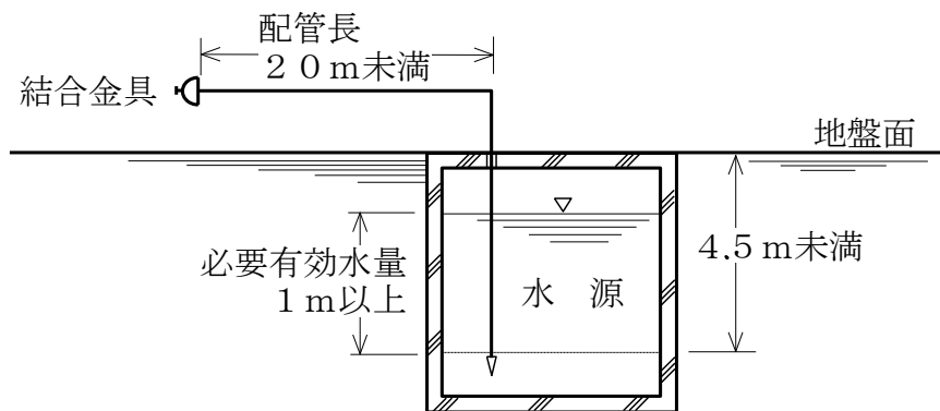
第18-1図 b 結合金具より下の水源を有する消防用水
