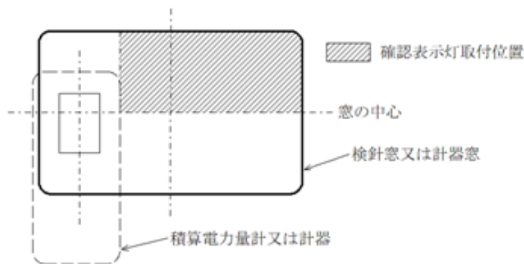
第24-1図 確認表示灯の取付け位置
