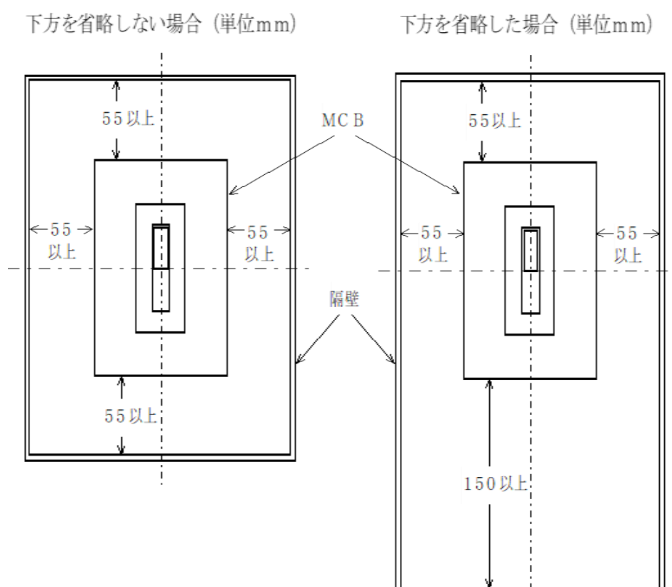
第24-2図 a 配線用遮断器と隔壁の離隔距離
