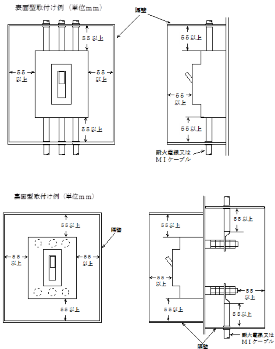
第24-2図 b 配線用遮断器の取付け例
