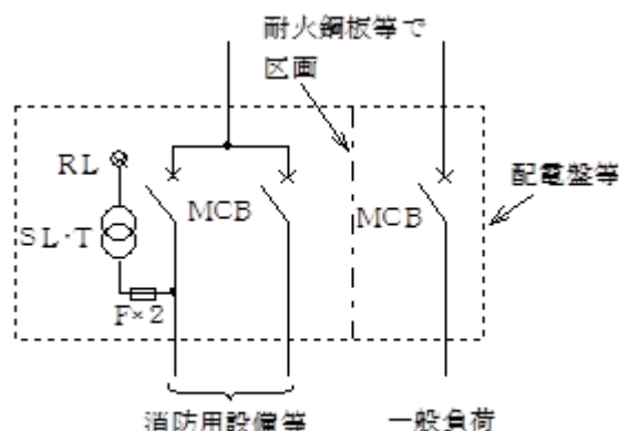
第24-3 図 b 配線の途中に使用する場合
