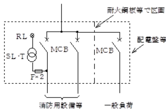
第24-3図 a 電力会社よりの受電点に使用する場合
