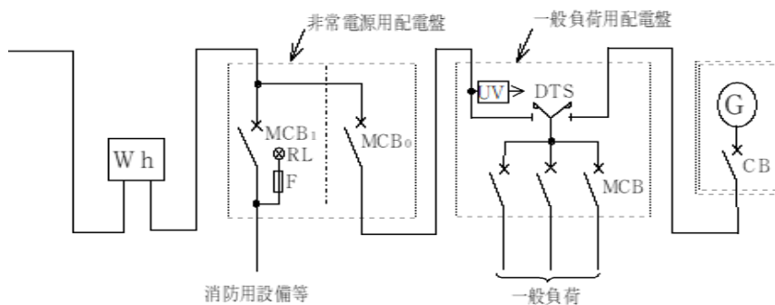
第24-7図 d ( 低圧で受電する場合)
