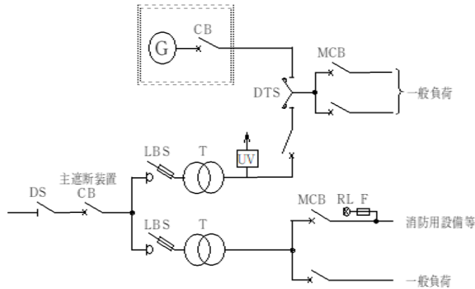
第24-7図 c ( 高圧又は特別高圧で受電する場合)
