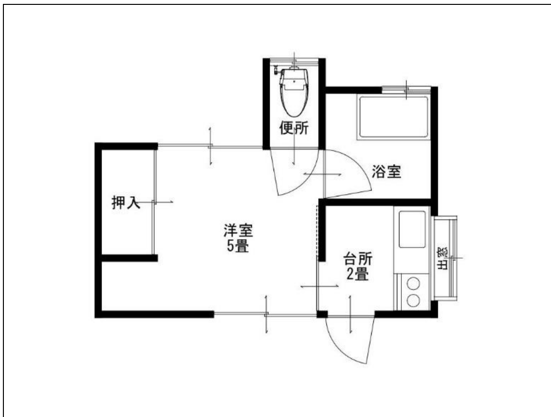
間取り図
