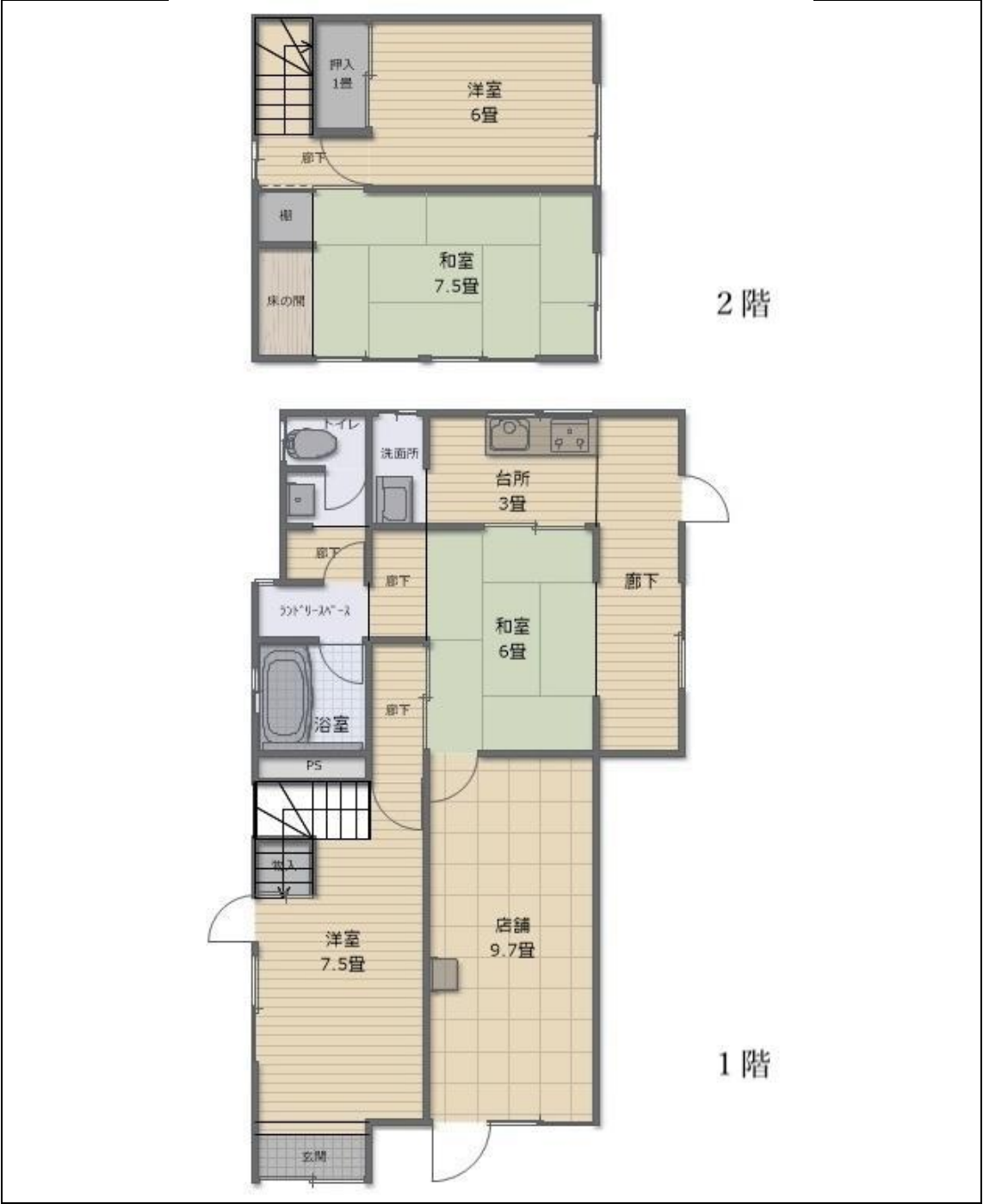
間取り図
